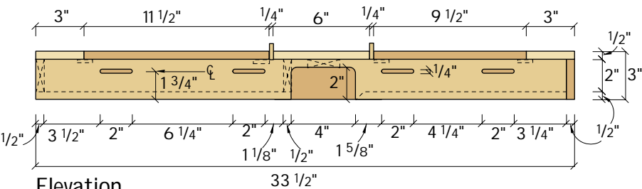
Elevation
